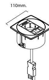
Tafelmodel Modèle pour table
