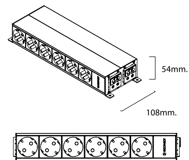
PDC enkel met voeding PDC simple avec alimentation.
