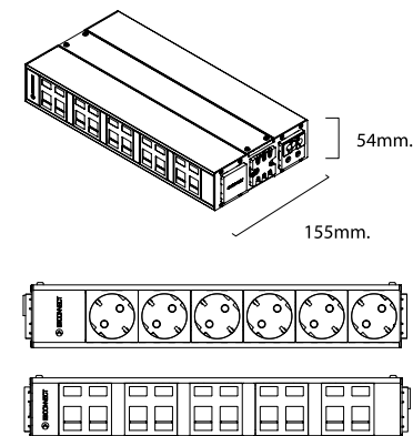
PDC met voeding en data PDC avec alimentation et data
