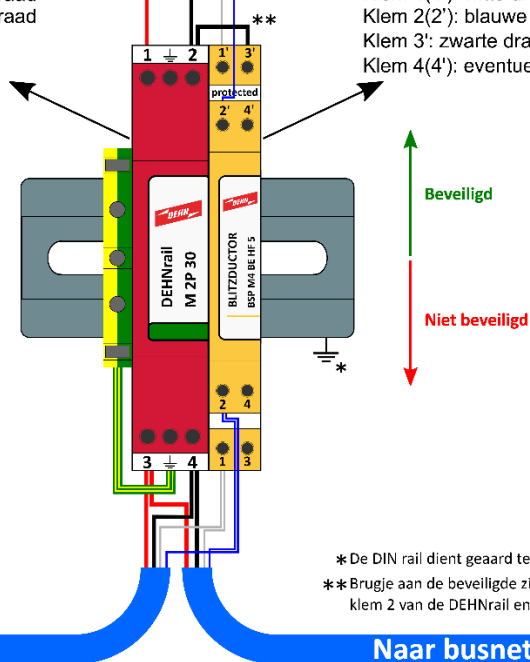
Figuur 4: principe schema voor het beveiligen van de AUTOBUS (dubbele aansluiting)
