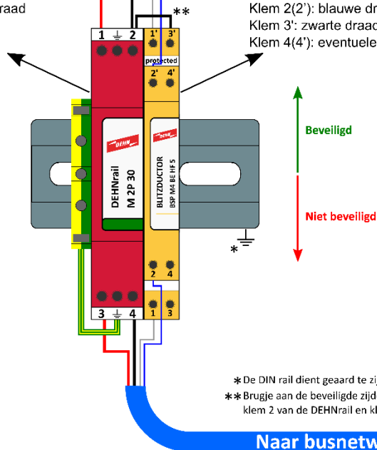
Figuur 3: principe schema voor het beveiligen van de AUTOBUS (enkele aansluiting)
