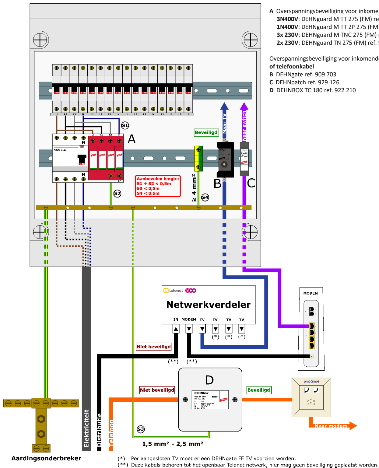
Figuur 2: aansluitschema beveiliging voor 230V, telefoonkabel en distributiekabel
