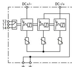
Schéma de principe du circuit DCB YPV 1500 FM
