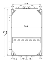
Dimensions IGA 10 V2 IP54
