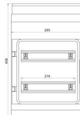
Dimensions IGA 24 IP54
