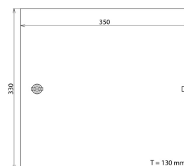
Dimensions DPG LSA 120 P
