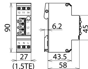
Dimensions DSI E 3
