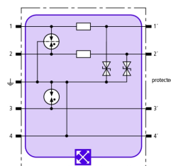
Schéma de principe du circuit BXT ML2 BE S 12
