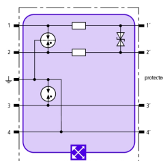
Schéma de principe du circuit BXT ML2 BD S 12
