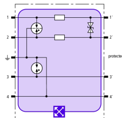
Schéma de principe du circuit BXT ML2 BD S 24
