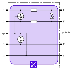
Schéma de principe du circuit BXT ML2 BD S 48
