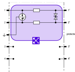
Schéma de principe du circuit BXT ML2 BD 180
