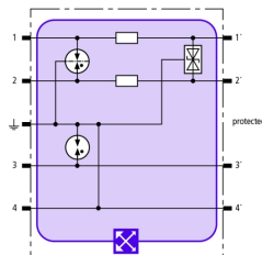
Schéma de principe du circuit BXT ML2 BE HFS 5
