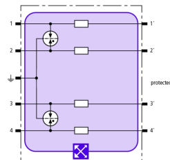
Schéma de principe du circuit BXT ML4 B 180
