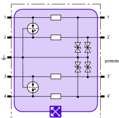
Schéma de principe du circuit BXT ML4 BE 12
