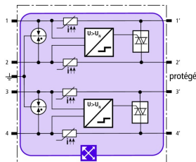
Schéma de principe du circuit BXTU ML4 BD 0-180
