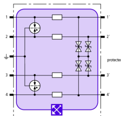
Schéma de principe du circuit BXT ML4 BC 5
