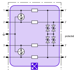
Schéma de principe du circuit BXT ML4 BC 24
