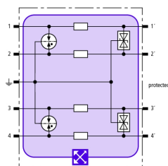
Schéma de principe du circuit BXT ML4 BE HF 5
