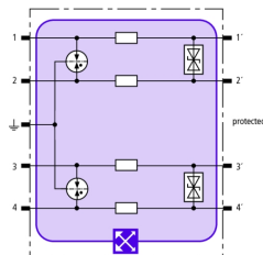
Schéma de principe du circuit BXT ML4 BD HF 24
