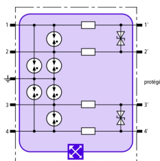
Schéma de principe du circuit BXT ML4 BD EX 24
