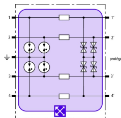
Schéma de principe du circuit BXT ML4 BC EX 24
