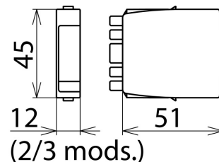
Dimensions BXT ML4 BC EX 24
