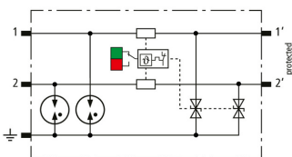
Circuit du BCO MOD ML2 BE 48
