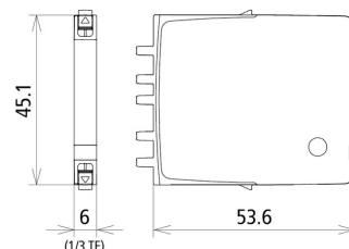
Dimension du BCO MOD ML2 BD 24
