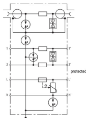
Schéma de principe du circuit DVR BNC RS485 230
