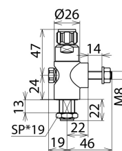
*) SP = Largeur sur pans
