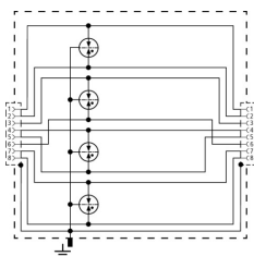
Schéma de principe du circuit DPA M CLD RJ45B 48
