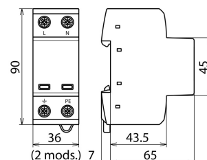
Dimensions DSH TT 2P 255
