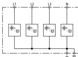
Schéma de principe du circuit DSH TNS 255
