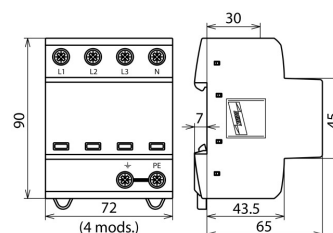
Dimensions DSH TNS 255
