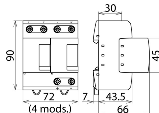
Dimensions DV M TT 2P 255
