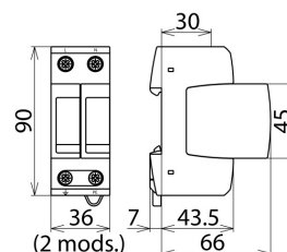
Dimensions DG M TT 2P 275
