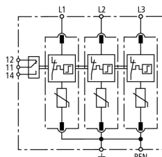
Schéma de principe du circuit DG M TNC 150 FM
