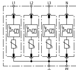
Schéma de principe du circuit DG M TNS 275
