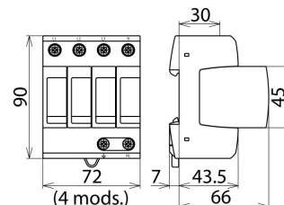
Dimensions DG M TNS 275
