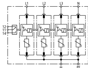
Schéma de principe du circuit DG M TNS 150 FM
