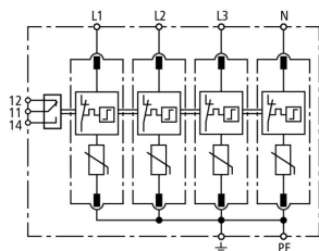
Schéma de principe du circuit DG M TNS 385 FM
