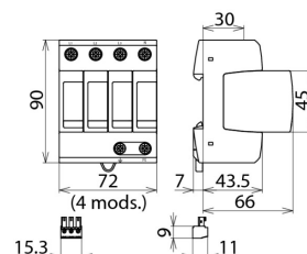
Dimensions DG M TNS 385 FM
