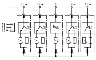
Schéma de principe du circuit DG M PV2 SCI 1000 FM
