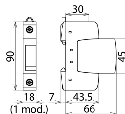
Dimensions DK 25
