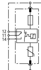
Schéma de principe du circuit DG S CI 440 FM
