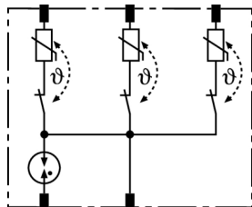
Schéma de principe du circuit DR MOD 4P 255
