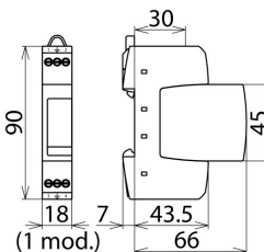
Dimensions DR M 2P 255
