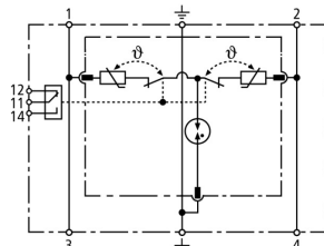
Schéma de principe du circuit DR M 2P 255 FM
