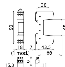
Dimensions DR M 2P 60 FM
