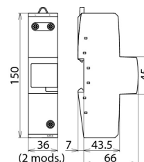
Dimensions DBM 1 440
