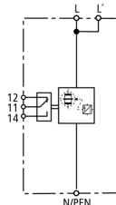
Schéma de principe du circuit DBM 1 440 FM
