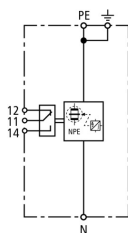
Schéma de principe du circuit DGPM 1 255 FM
