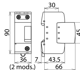
Dimensions DSE M 1 60
