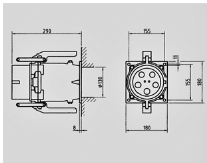
Schéma 2 MB 199/1
