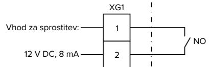
sl. 12: Osnovna vezalna shema: priključitev zunanega preklopnega kontakta
