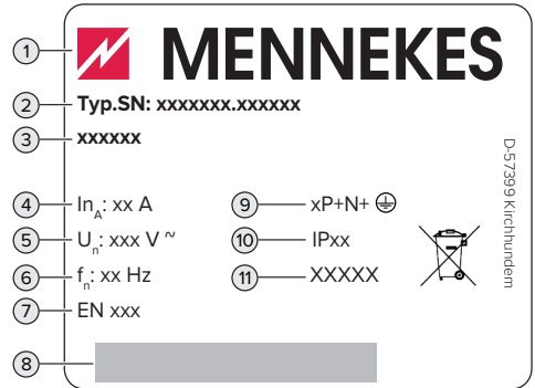
Afb. 1: Typeplaatje (monster)
