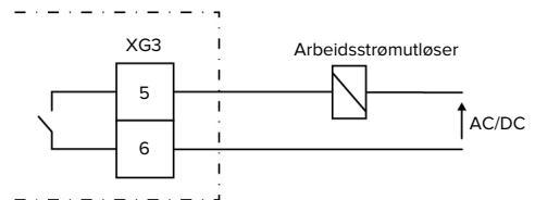
Fig. 8: Prinsipielt koblingsskjema: tilkobling av ekstern arbeidsstrømutløser
