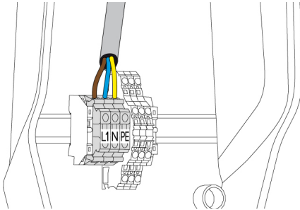
Abb. 7: Anschluss Spannungsversorgung
