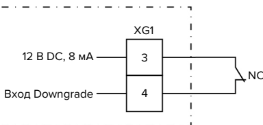
Рис. 11: Принципиальная схема: подключение внешнего переключающего контакта
