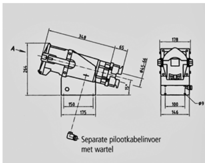
Tekening 1 MB 385
