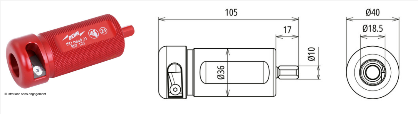
Tête de fraisage pour conducteur HVI light plus.
